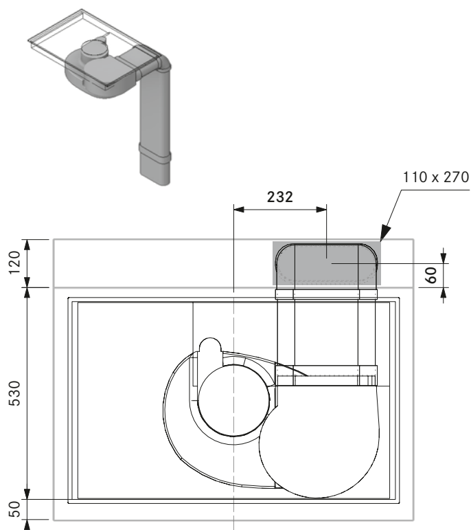
Mindestmaß Kernbohrung PUXA mit Flachkanal EF750 (Insel; Tiefe 700):
