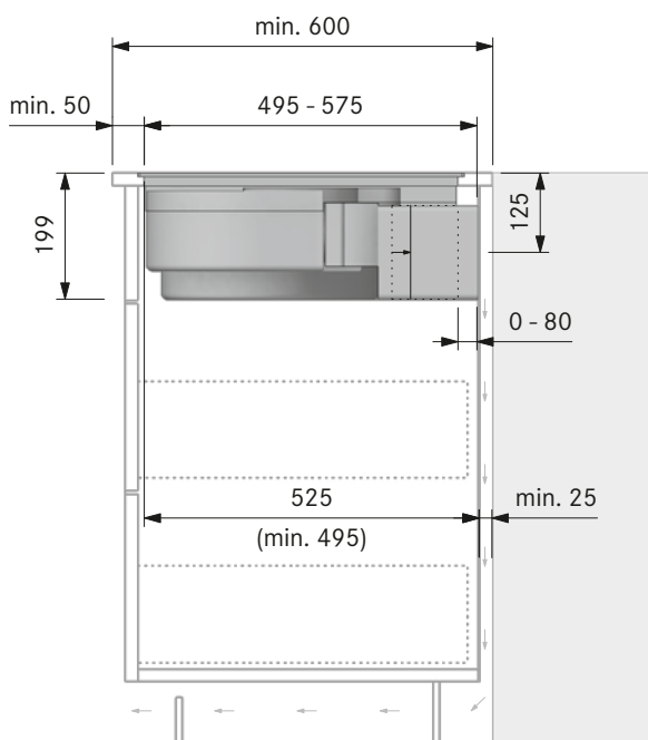
Einbauschnitt PURU (Zeile 600):
