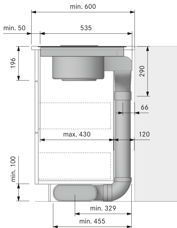
Einbauschnitt Basic Abluft (Zeile 600):
