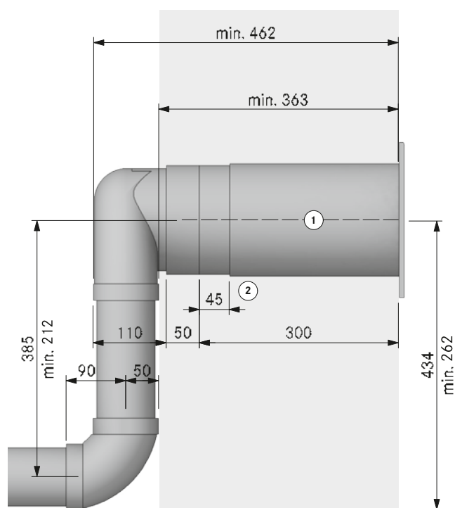
MP_9062 Kanalführung mit S-Kurve Mauerkasten UEBR
