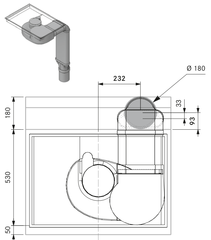
Mindestmaß Kernbohrung PURA mit Flachkanal EF750, Übergangsstück gerade EFRG (Insel):
