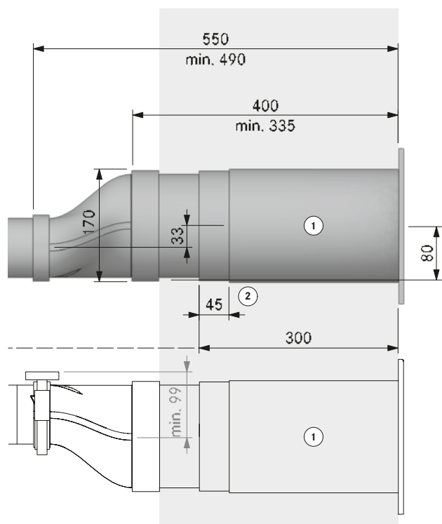
MP_9066 Kanalführung flach mit Übergang auf Mauerkasten UEBR
