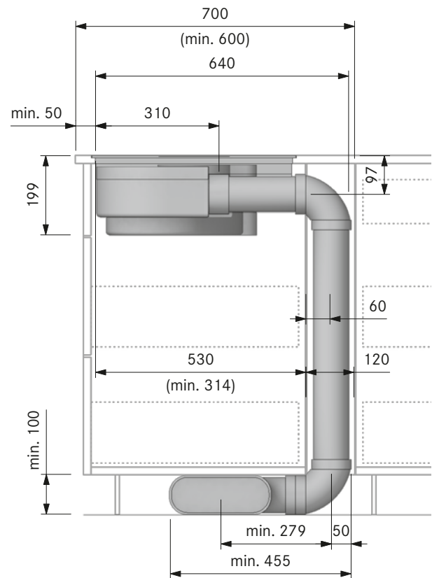
Einbauschnitt PURA Abluft (Insel):
