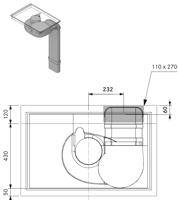
Mindestmaß Kernbohrung PUXA mit Flachkanal EF750 (Zeile; Tiefe 600):
