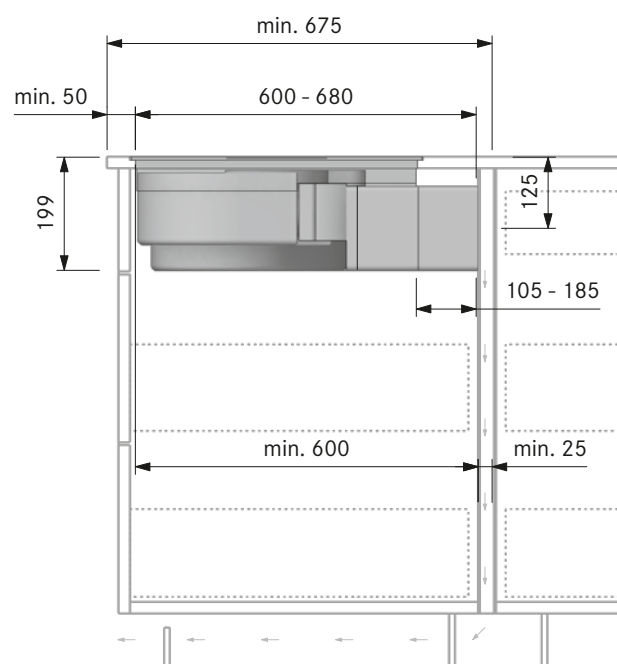
Einbauschnitt PURU mit zusätzlichem Teleskopauszug PULBTA (Insel):
