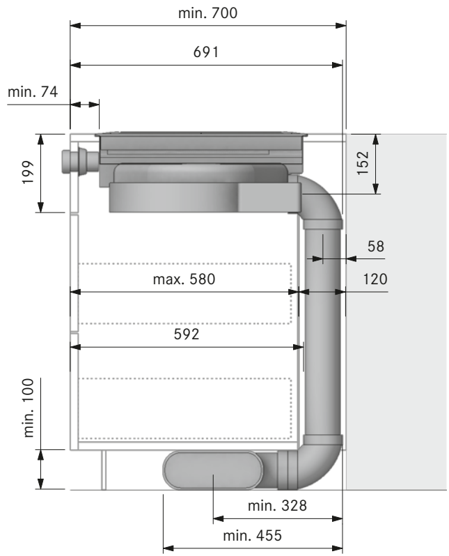
PKAS3 mit Ecotube Flachkanal:
