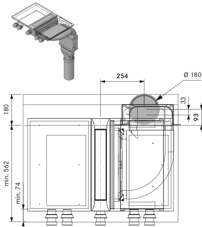
Mindestmaß Kernbohrung PKA3 mit Flachschalldämpfer USDF und Übergangsstück gerade EFRG (Insel):
