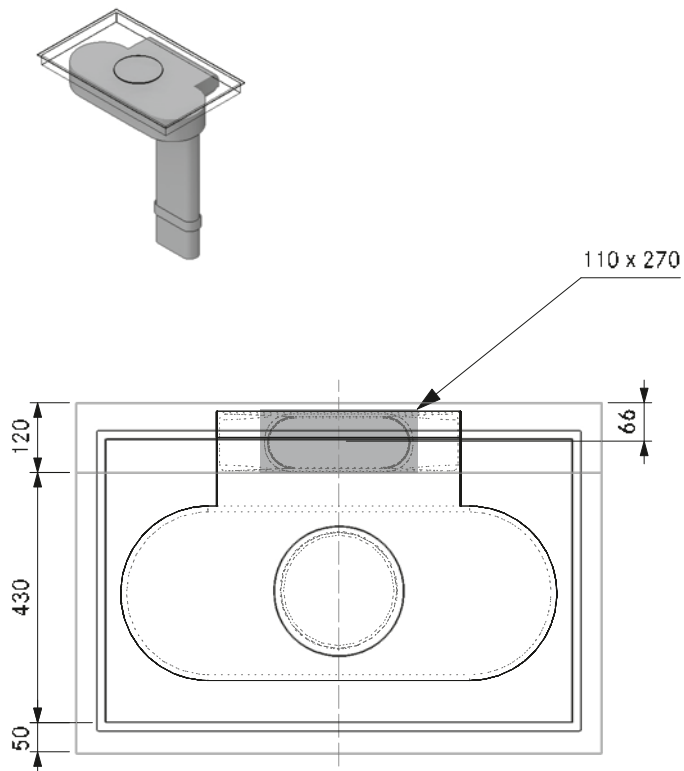
Mindestmaß Kernbohrung Basic mit Flachkanal EF750 (Tiefe 600):
