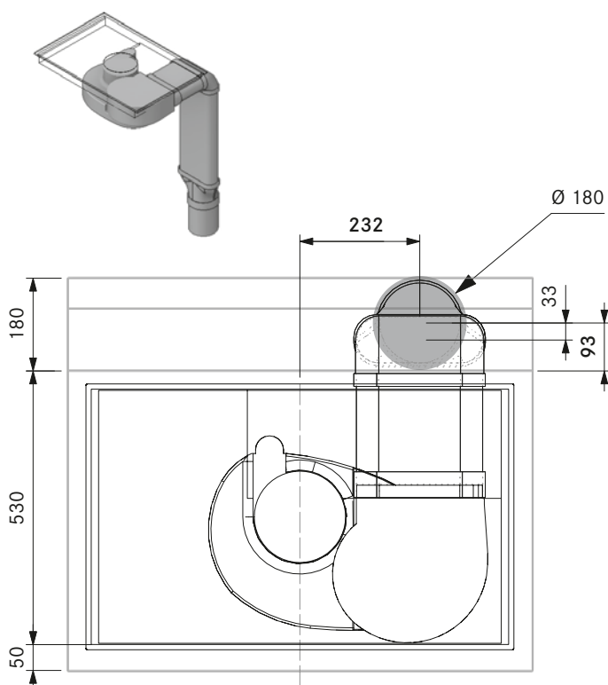
Mindestmaß Kernbohrung PUXA mit Flachkanal EF750, Übergangsstück gerade EFRG (Insel):
