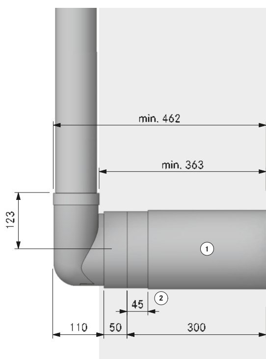
MP_9068 Kanalführung hochkant mit Übergang EFR90 auf Mauerkasten UEBR
