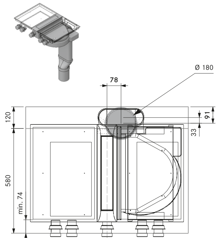
Mindestmaß Kernbohrung PKA3 mit Flachkanal EF750 und Übergangsstück gerade EFRG (Zeile):
