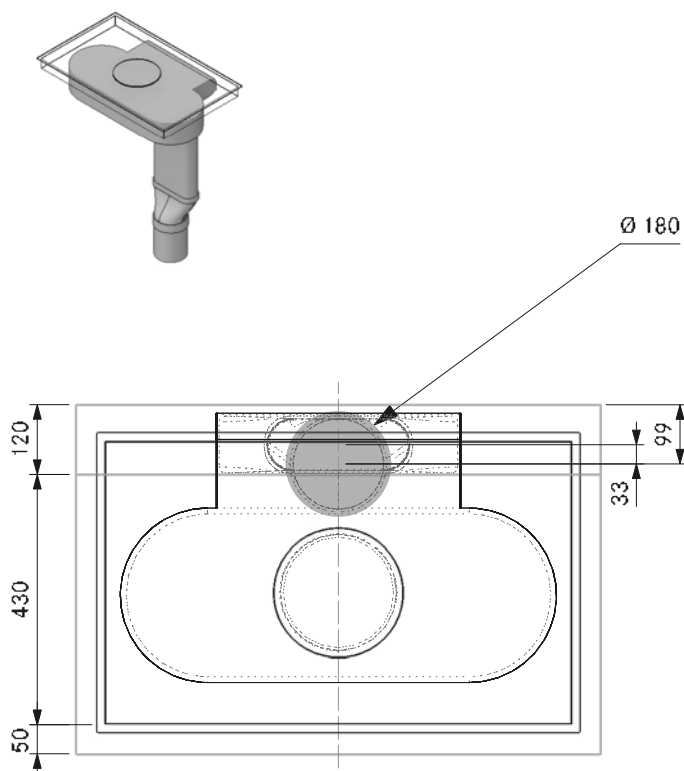
Mindestmaß Kernbohrung Basic mit Flachkanal EF750, Übergangsstück gerade EFRG (Zeile):
