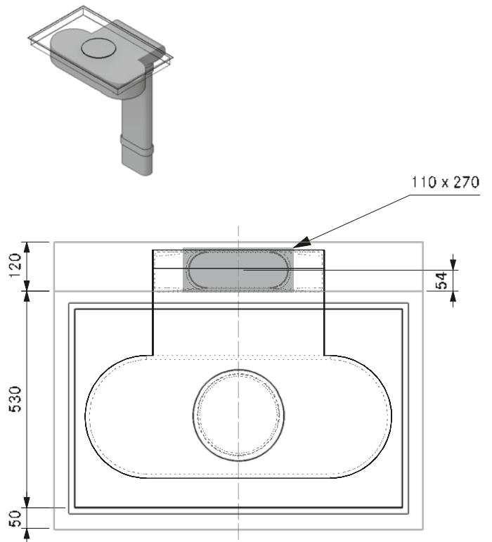
Mindestmaß Kernbohrung Basic mit Flachkanal EF750 (Tiefe 700):
