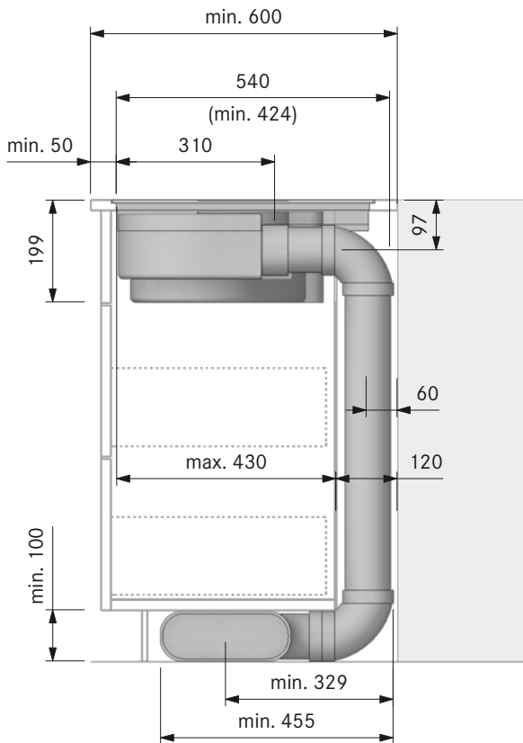
Einbauschnitt PURA Abluft (Zeile 600):
