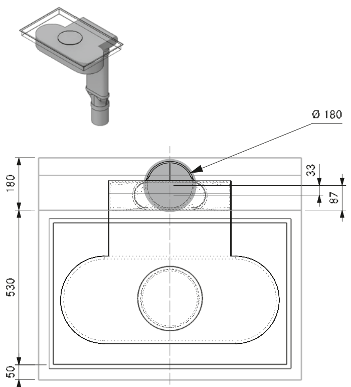
Mindestmaß Kernbohrung Basic mit Flachkanal EF750, Übergangsstück gerade EFRG (Insel):
