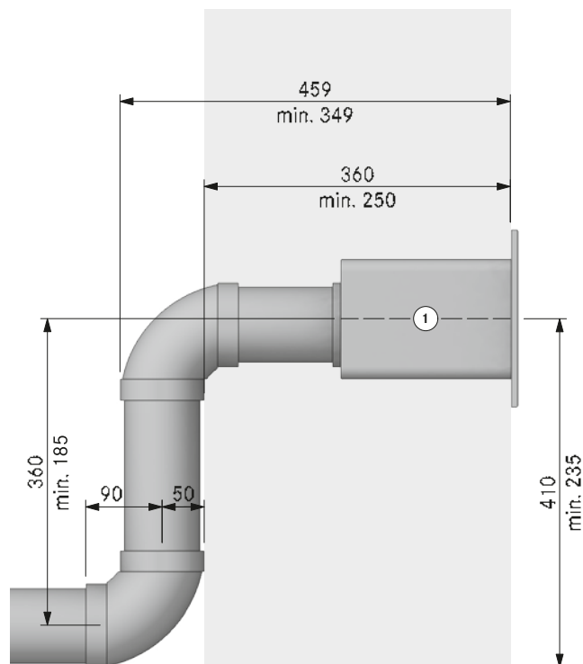
MP_9042 Kanalführung mit S-Kurve Mauerkasten UEBF
