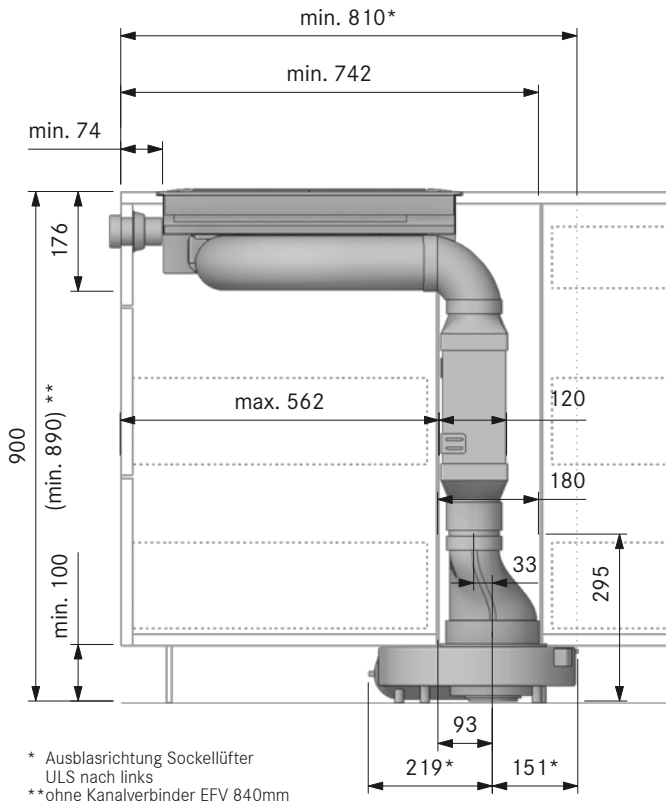
PKA3 mit Rundschalldämpfer USDR50 und Rundkanalverbinder ERV (Insel):
