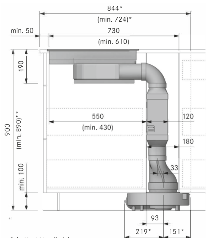
CKA2 mit Flachschalldämpfer USDF, Flachkanalverbinder EFV und Übergangsstück gerade EFRG (Insel):
