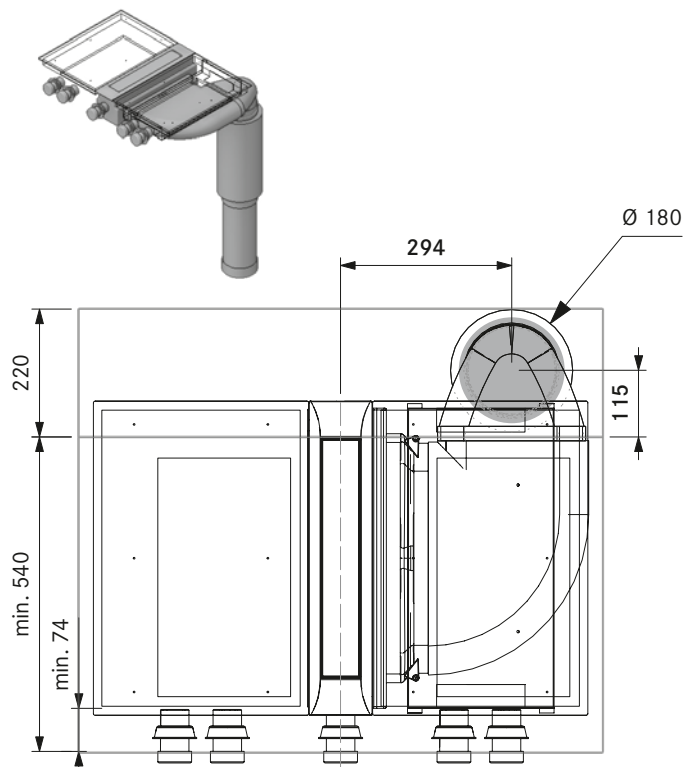
Mindestmaß Kernbohrung PKA3 mit Rundschalldämpfer USDR50 (Insel):
