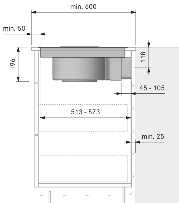
Einbauschnitt Basic Umluft (Zeile 600):
