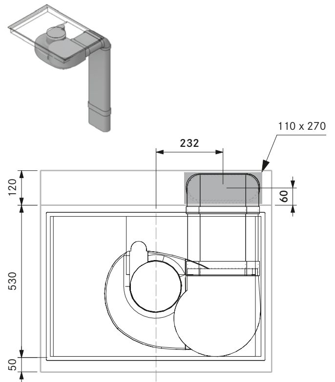
Mindestmaß Kernbohrung PURA mit Flachkanal EF750 (Insel; Tiefe 700):
