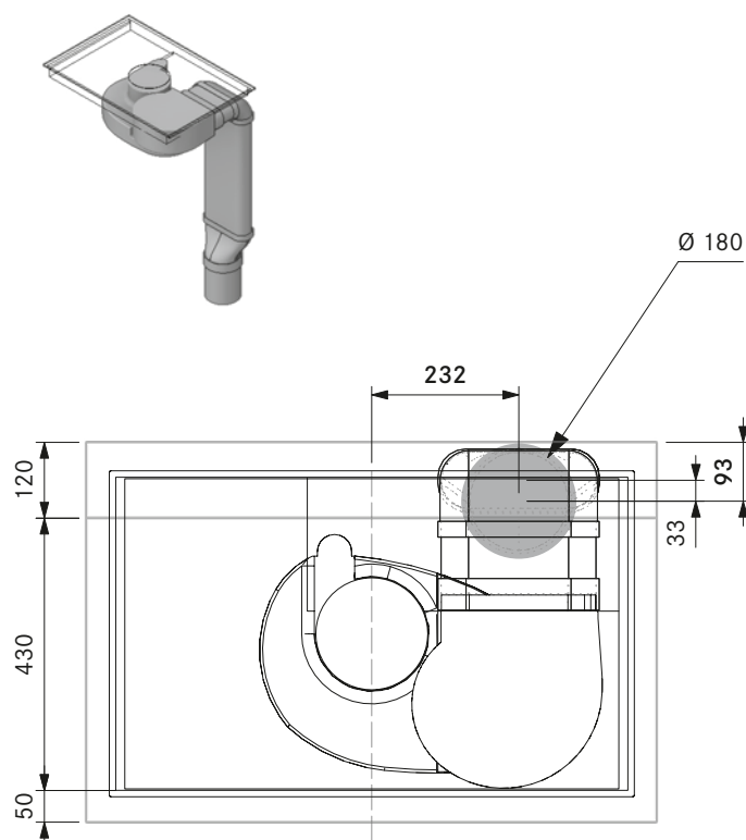
Mindestmaß Kernbohrung PUXA mit Flachkanal EF750, Übergangsstück gerade EFRG (Zeile):
