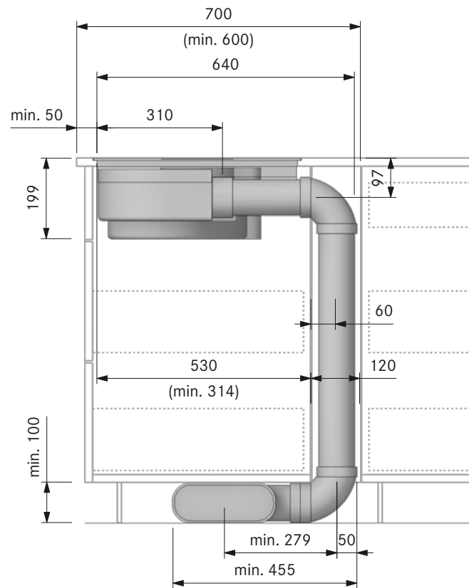
Einbauschnitt PUXA Abluft (Insel):
