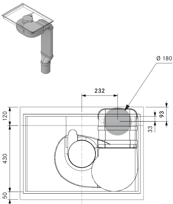
Mindestmaß Kernbohrung PURA mit Flachkanal EF750, Übergangsstück gerade EFRG (Zeile):
