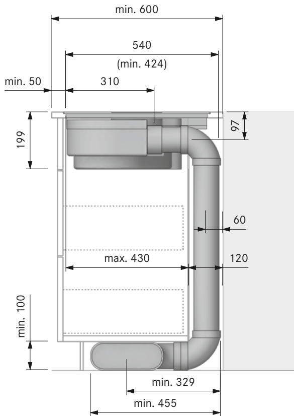
Einbauschnitt PUXA Abluft (Zeile 600):
