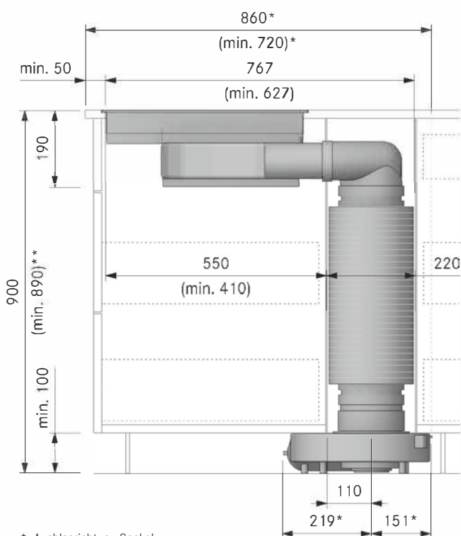
CKA2 mit Rundschalldämpfer USDR50 und Rundkanalverbinder ERV (Insel):
