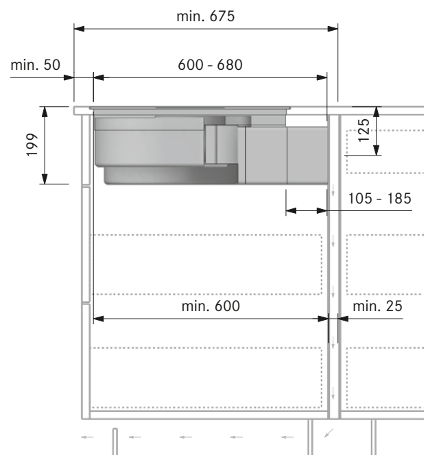
Einbauschnitt PUXU mit zusätzlichem Teleskopauszug PULBTA (Insel):
