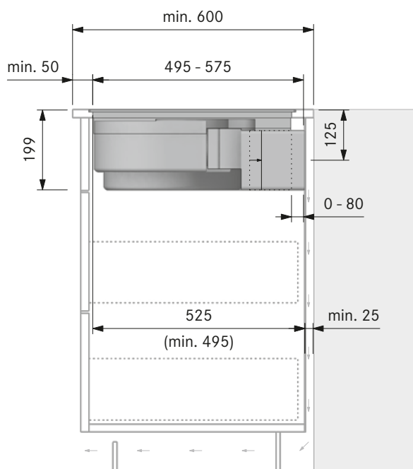
Einbauschnitt PUXU (Zeile 600):
