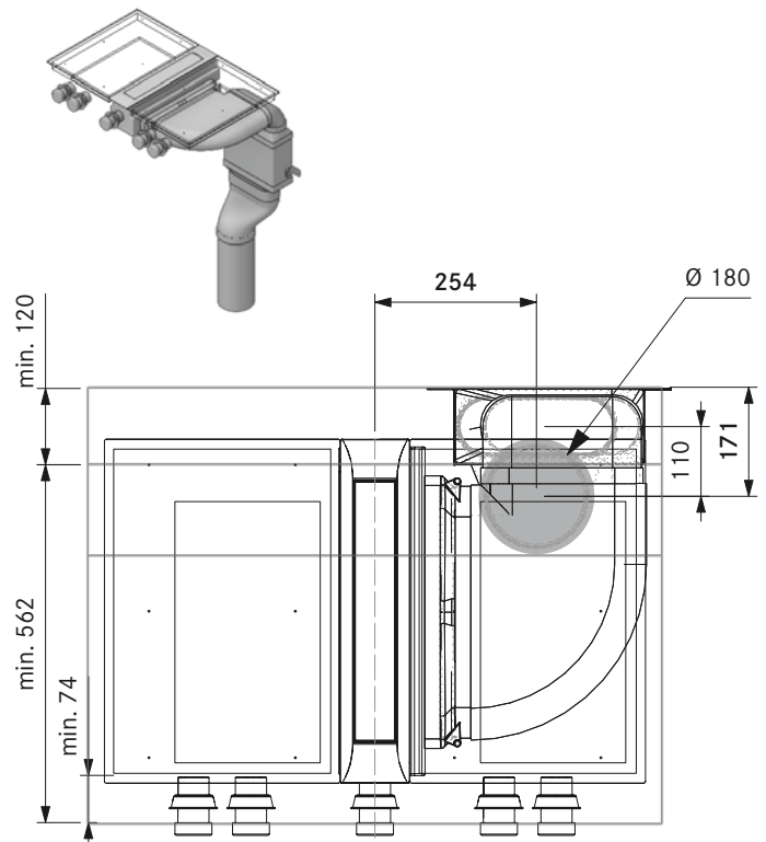
Mindestmaß Kernbohrung PKA3 mit Flachschalldämpfer USDF und Übergangsstück Versatz EFRV110 (Zeile):
