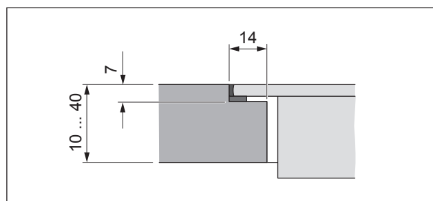
Abb. 5.4 Falzmaß für flächenbündige Montage
