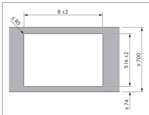
Abb. 5.5 Aufsatzmontage
