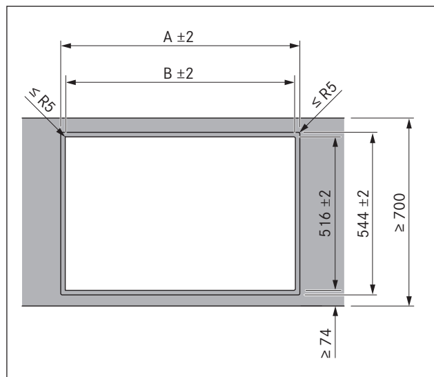
Abb. 5.3 Flächenbündige Montage
