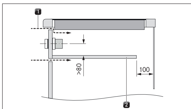
Abb. 5.7 Luftzufuhr über den Frontbereich
