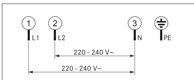
Abb. 5.22 Anschlusschema 2-phasig
