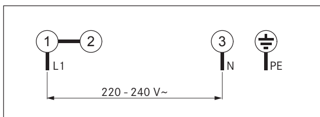
Abb. 5.23 Anschlusschema 1-phasig
